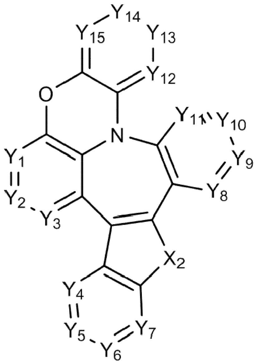
[화학식 5]
