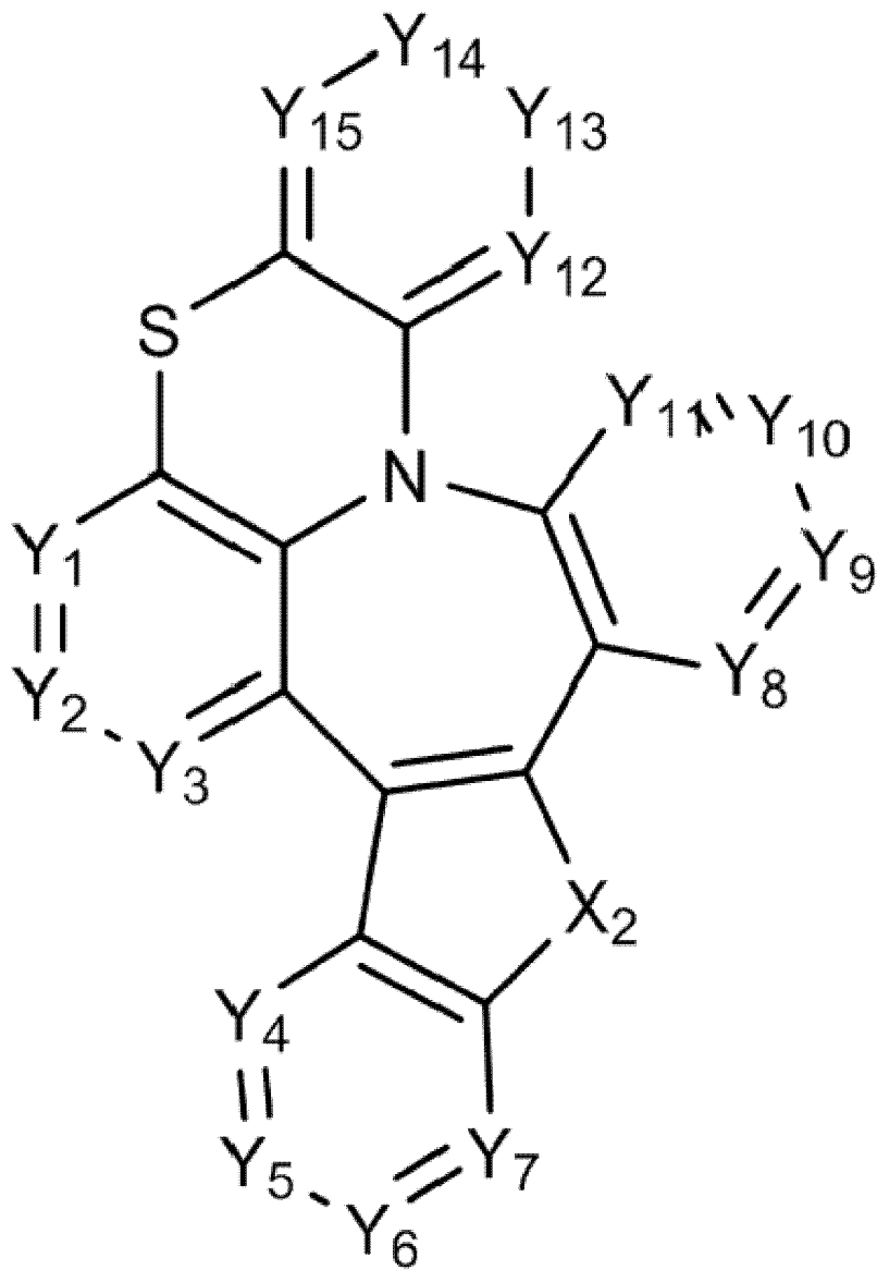
[화학식 6]
