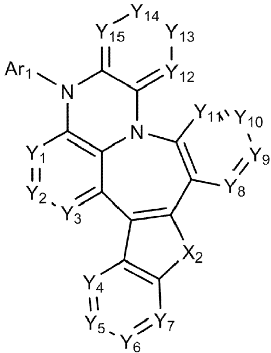
[화학식 7]
