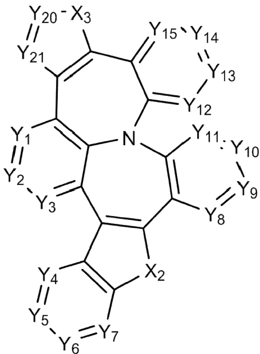
[화학식 12]
