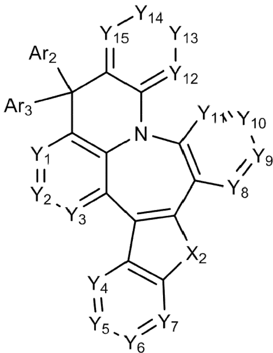
[화학식 8]
