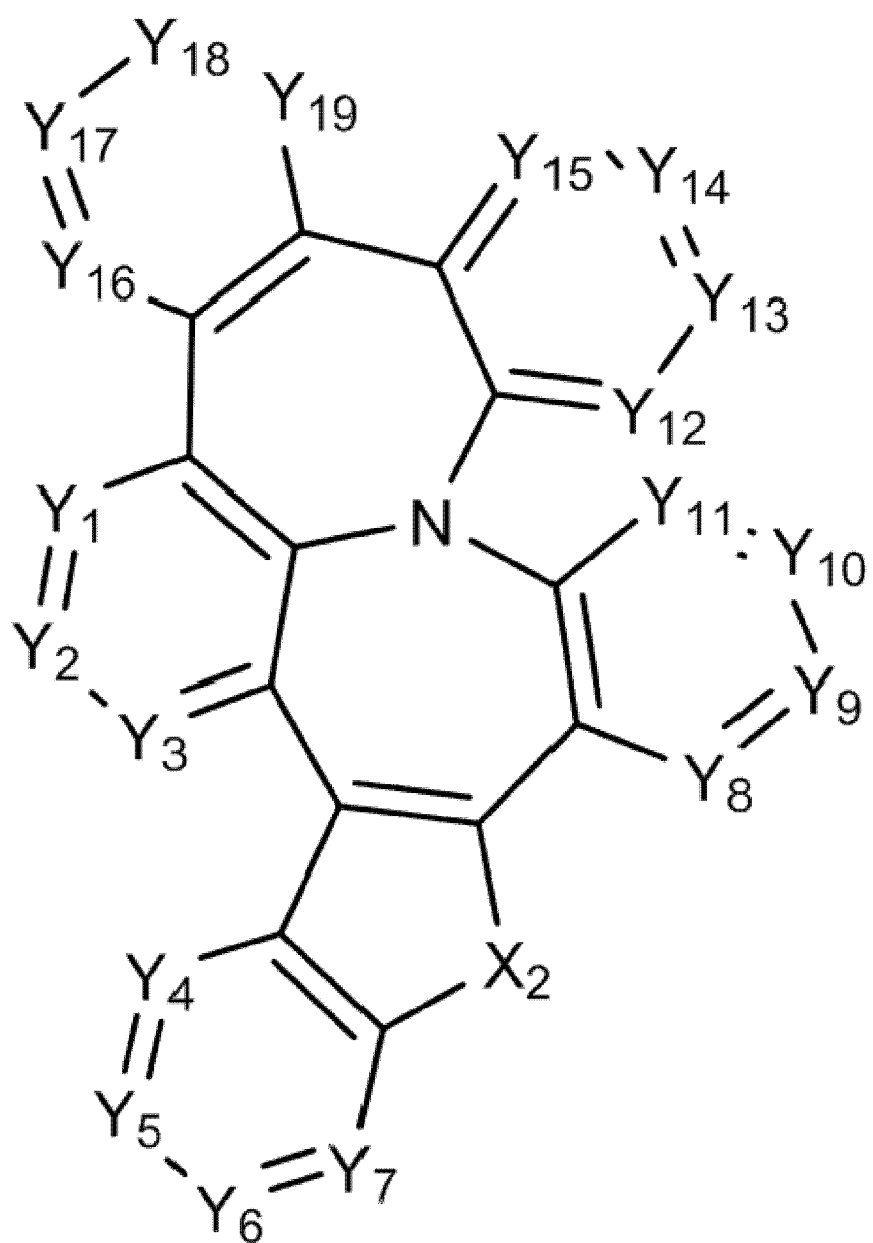
[화학식 11]
