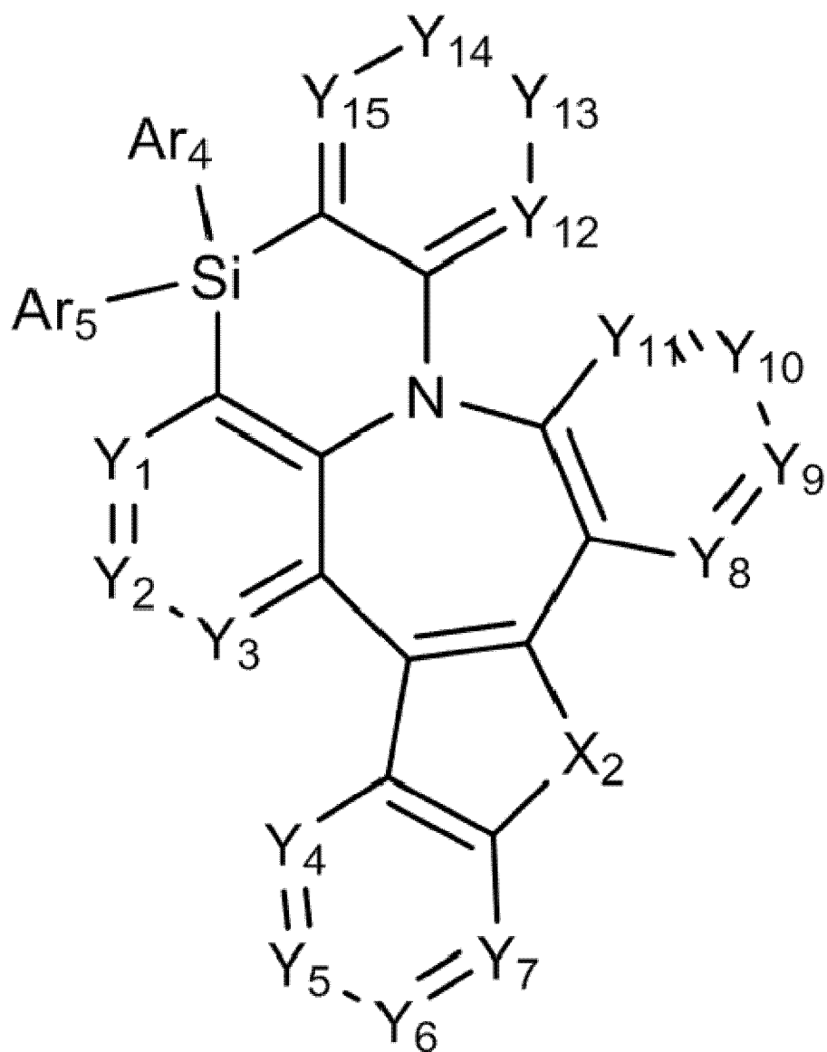
[화학식 9]
