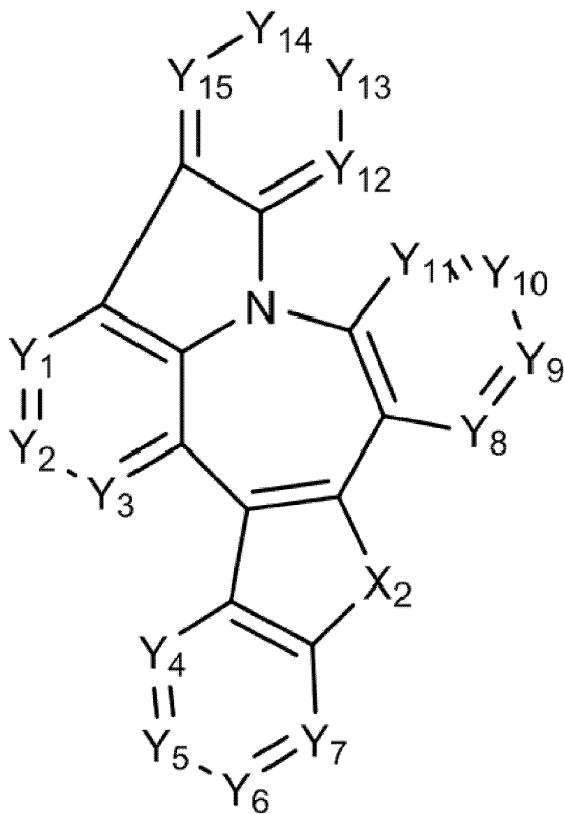
[화학식 4]
