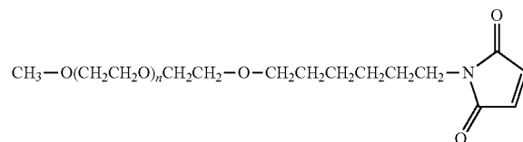
mPEG-HEXA-MAL
