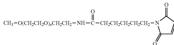
mPEG-AMPE-MAL
