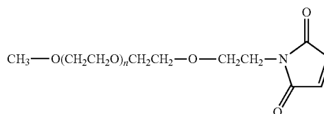
mPEG-ET-MAL
