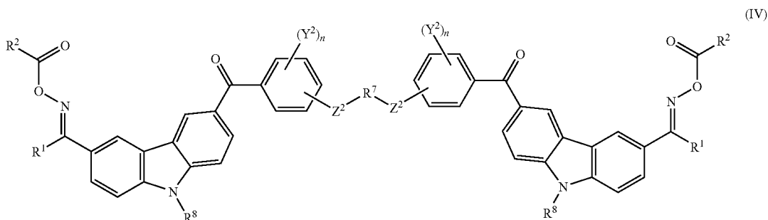
[Formula 38]
