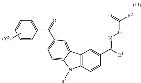
[Formula 37]
