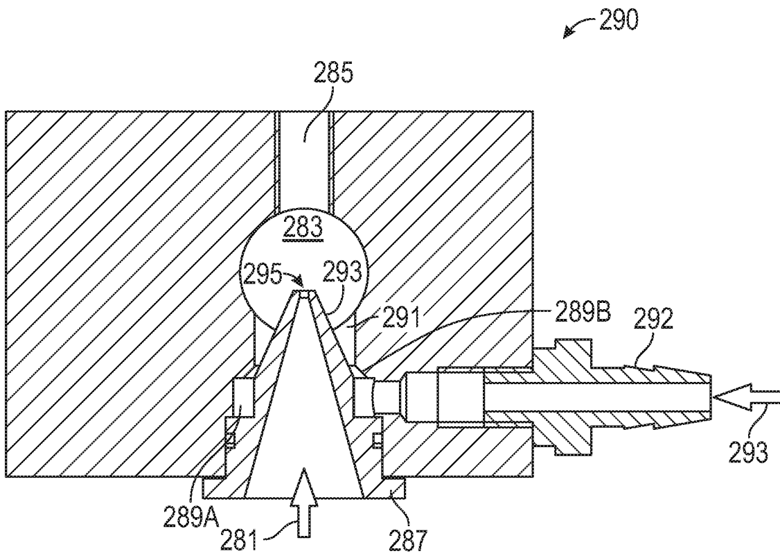
FIG. 2E SECTION A-A
