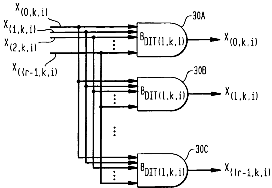
FIG. 5A JABER'S RADIX-r DIF MODULE
