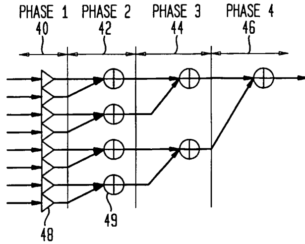
FIG. 6A RADIX-8 DIT FFT ENGINE
