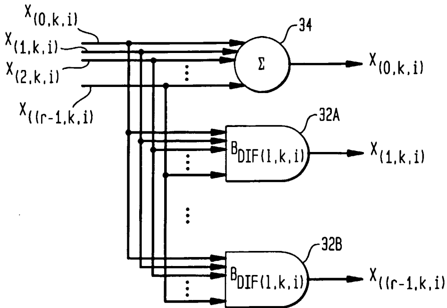
FIG. 5B JABER'S RADIX-r DIT MODULE
