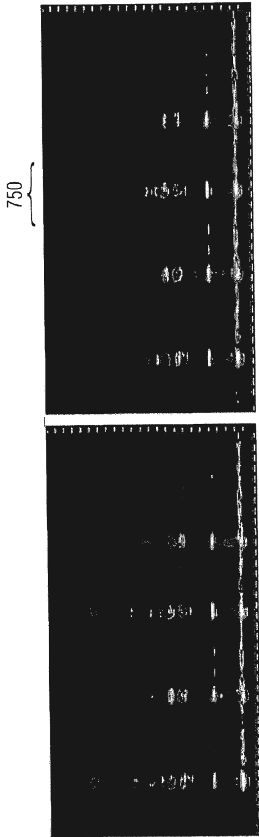
ESPECTROGRAMA DE TRANSFORMADA DISCRETA DE FOURIER (DFT) DE LA SEÑAL ORIGINAL (Panel Izquierdo); ESPECTROGRAMA DE DFT DE LA SEÑAL EXTENDIDA SIN TTS (Panel Derecho).
