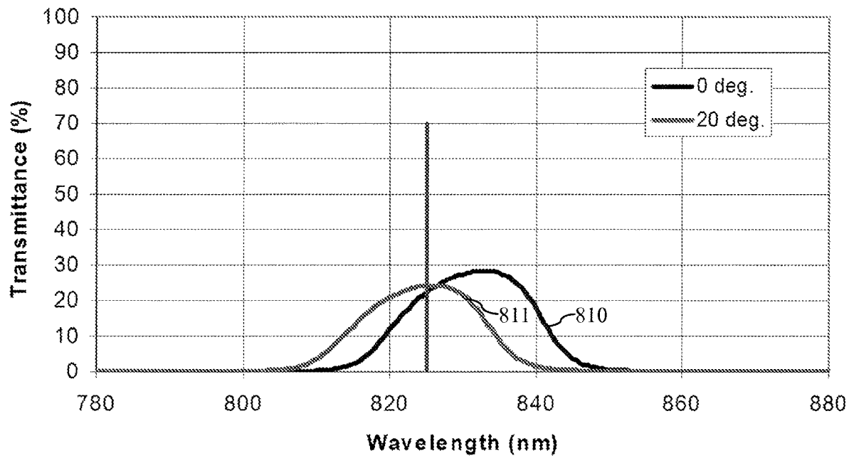
FIG. 8D
