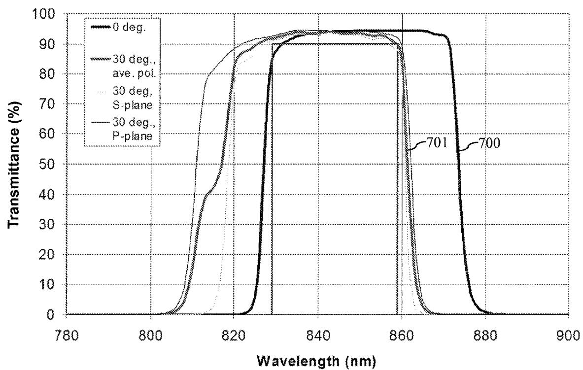
FIG. 7D
