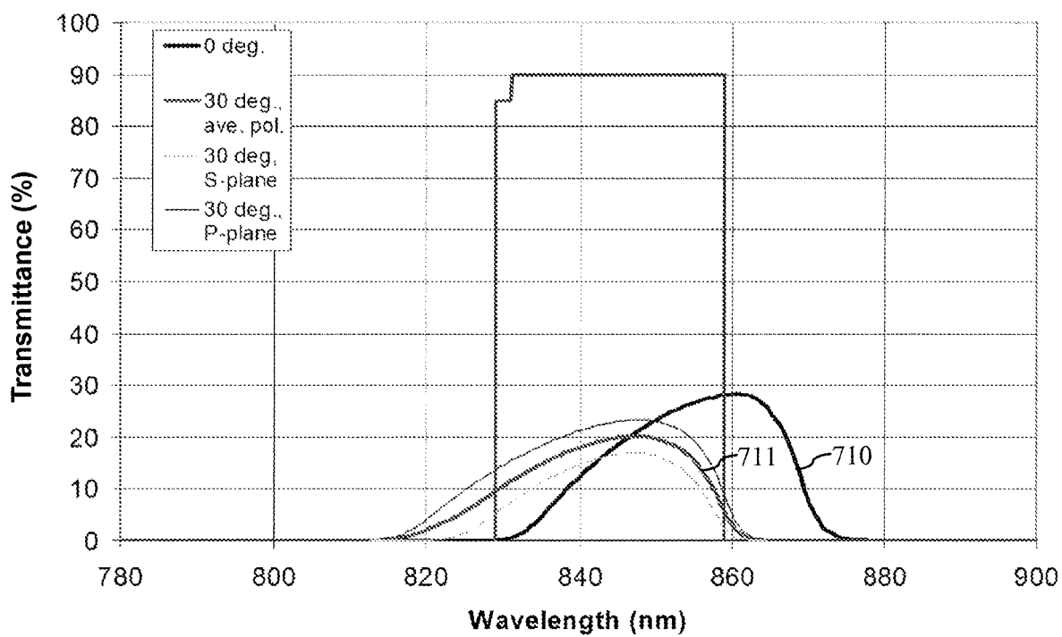
FIG. 7E
