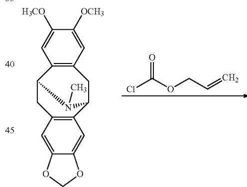
Scheme 26: (+)-Eschscholtzidine
