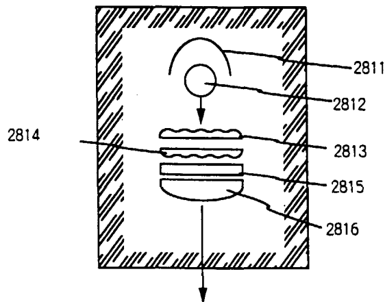
Fig. 18(D) Light Source Optical System
