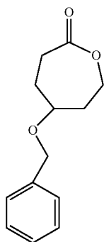
5-(Benzyloxy)oxepan-2-one (BXO)
