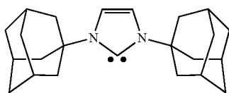
1,3-Bis(1-adamantyl)imidazol-2-ylidene (Im-4)
