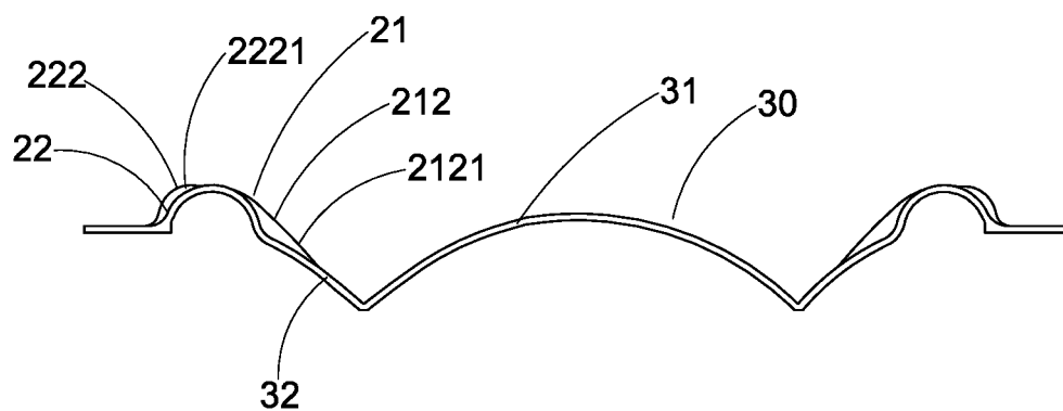
B-B FIG.14
