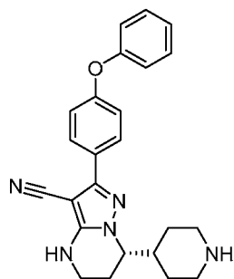
Formula 1e
