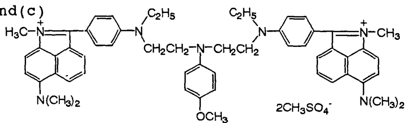
Compound (d)
