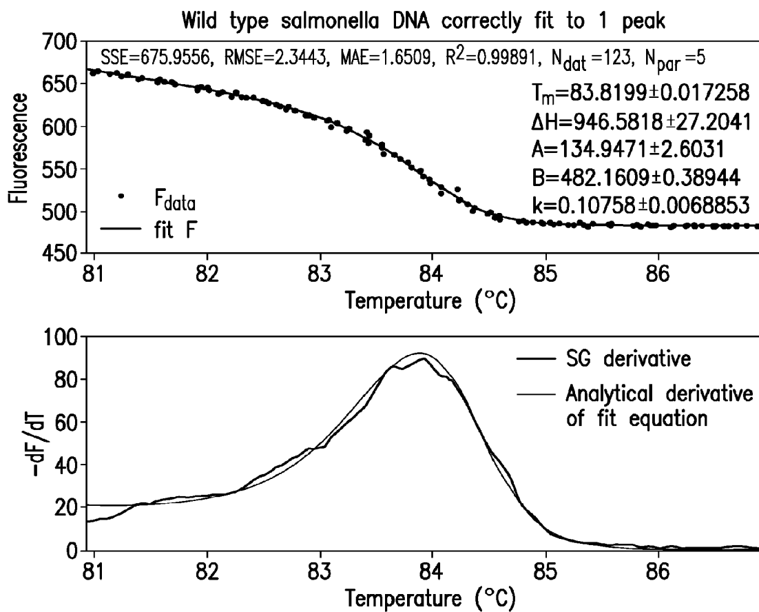
FIG. 7A
