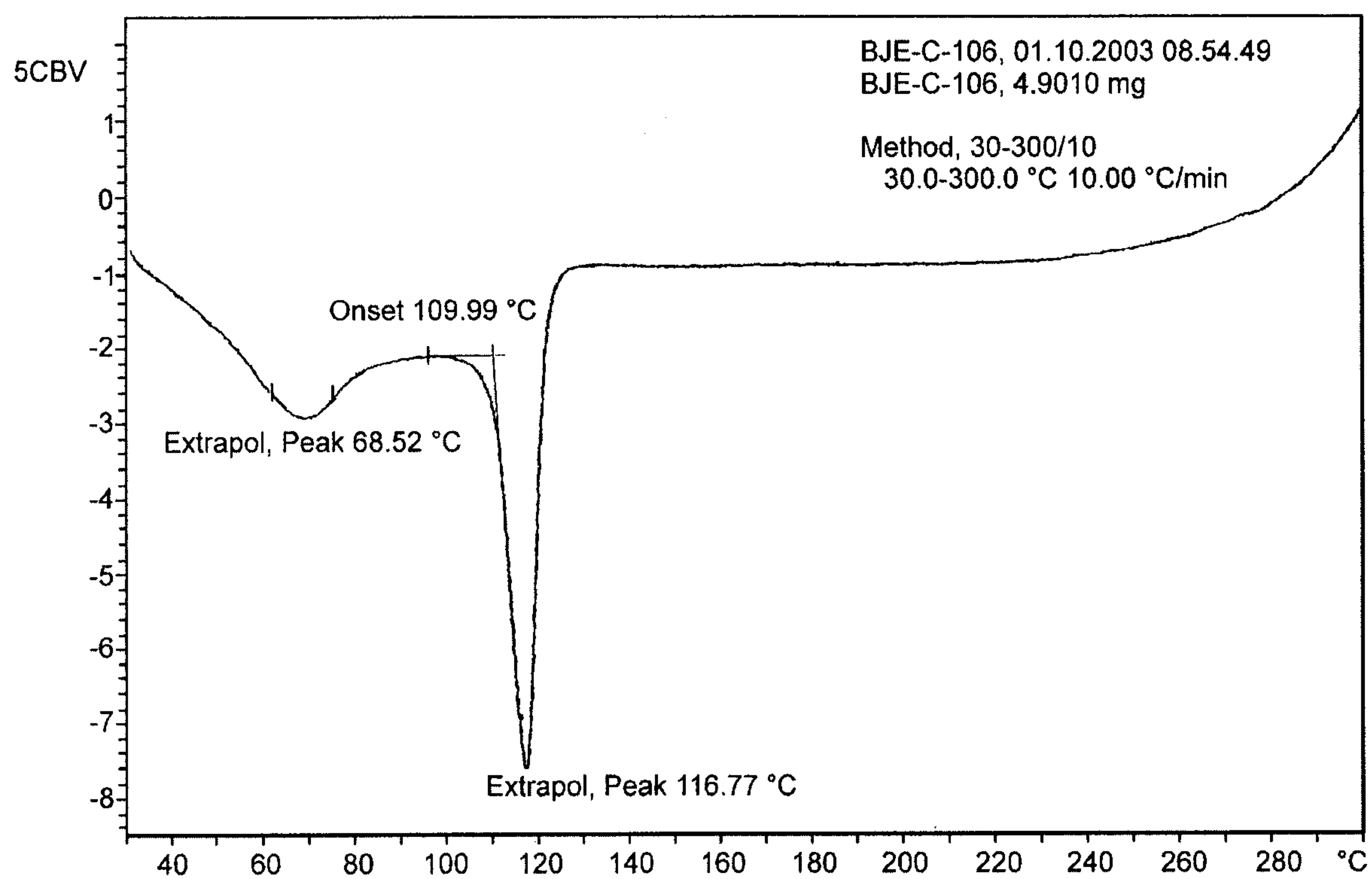
FIG. 5
