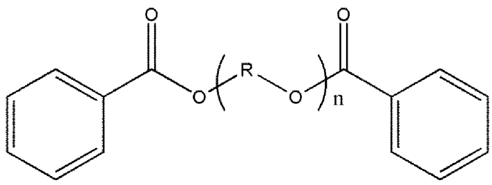
[Formule chimique 2]
