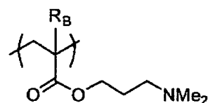
(B-18)
