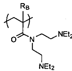
(B-27)
