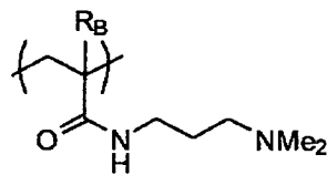
(B-24)
