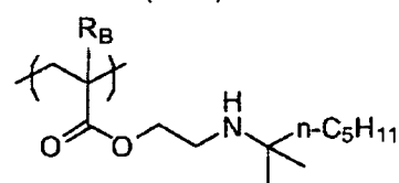
(B-35)
