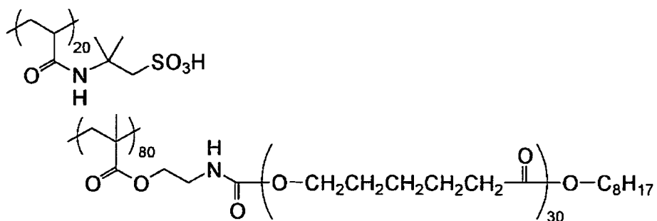
(B-1-5) Mw 42,000
