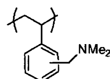
(B-20)
