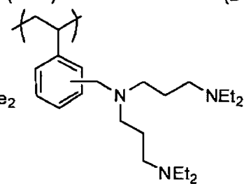
(B-31)
