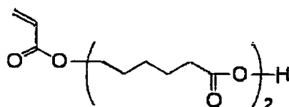
Monomer g
