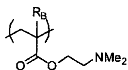
(B-14)
