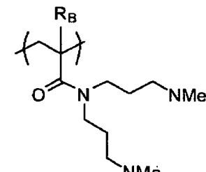
(B-28)
