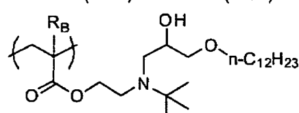
(B-36)
