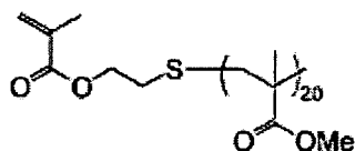
Macromonomer (1-3)
