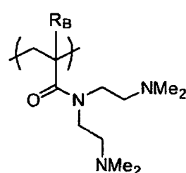
(B-26)
