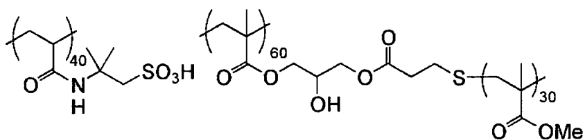
(B-1-7) Mw 36,000
