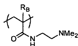
(B-22)
