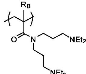
(B-29)
