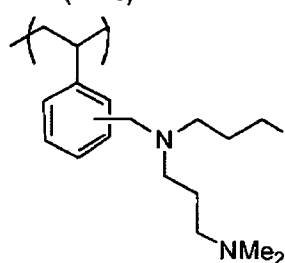
(B-30)
