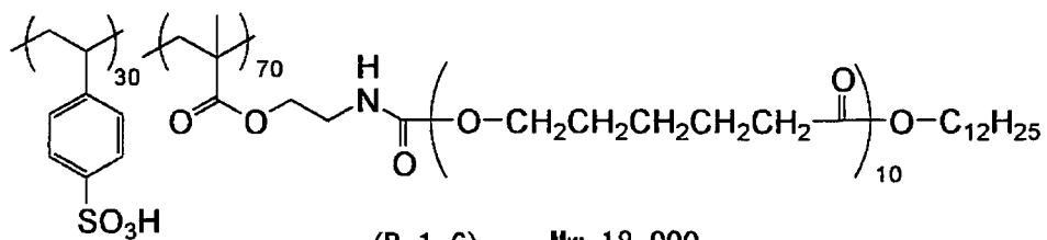
(B-1-6) Mw 18,000
