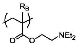
(B-15)
