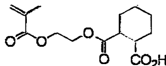
Monomer e
