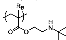
(B-34)
