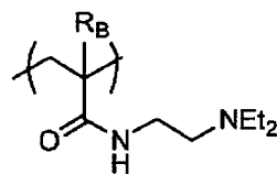
(B-23)
