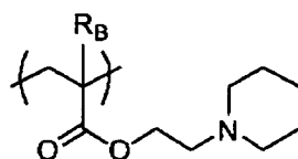
(B-16)
