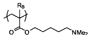
(B-19)
