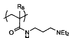
(B-25)
