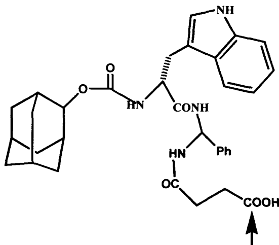
CI-988
