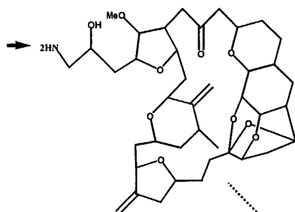
ER-086526
