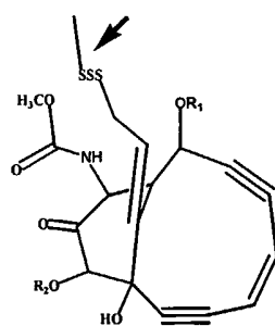
Esperamycin
