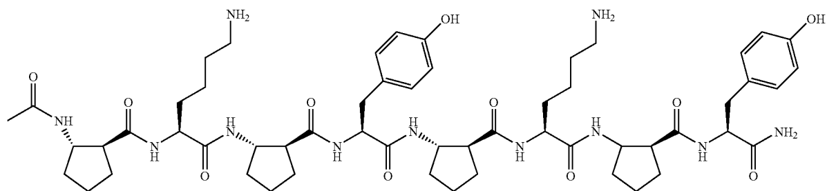
(S,S)-ACPC L-amino acids
