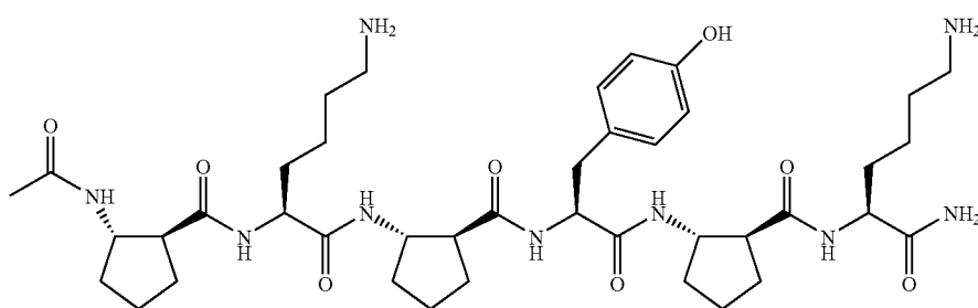
(S,S)-ACPC L-amino acids
