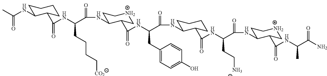
Ac-ACHC-E-PIP-Y-ACHC-K-PIP-A-NH 2 (S) ACHC, (S) PIP, (D) amino acids
