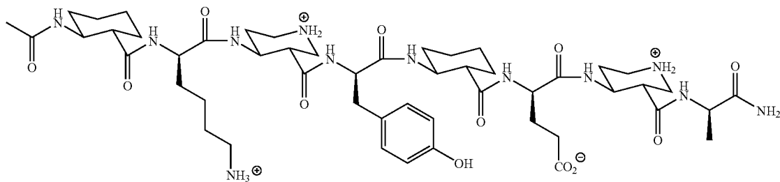
Ac-ACHC-K-PIP-Y-ACHC-E-PIP-A-NH 2 (S) ACHC, (S) PIP, (D) amino acids
