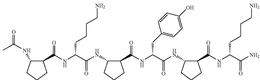
(S,S)-ACPC D-amino acids
