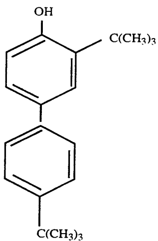
2-t-butyl-4-(4'-t-butylphenyl)phenol
