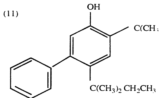
2-t-butyl-4-(1,1-dimethylpropyl)-5-phenylphenol
