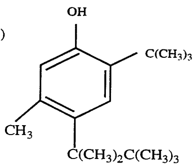
2-t-butyl-4-(1,1,2,2-tetramethylpropyl)-5-methylphenol
