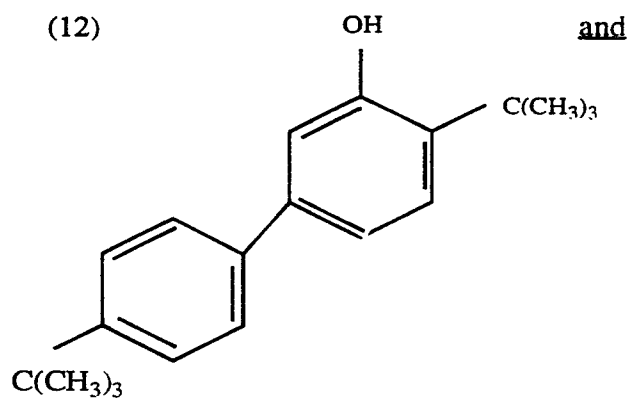
2-t-butyl-5-(4'-t-butyl-phenyl)phenol
