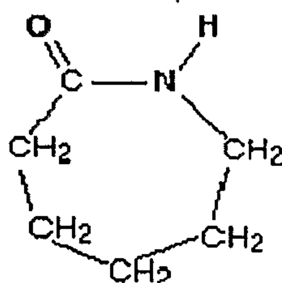
caprolactam
