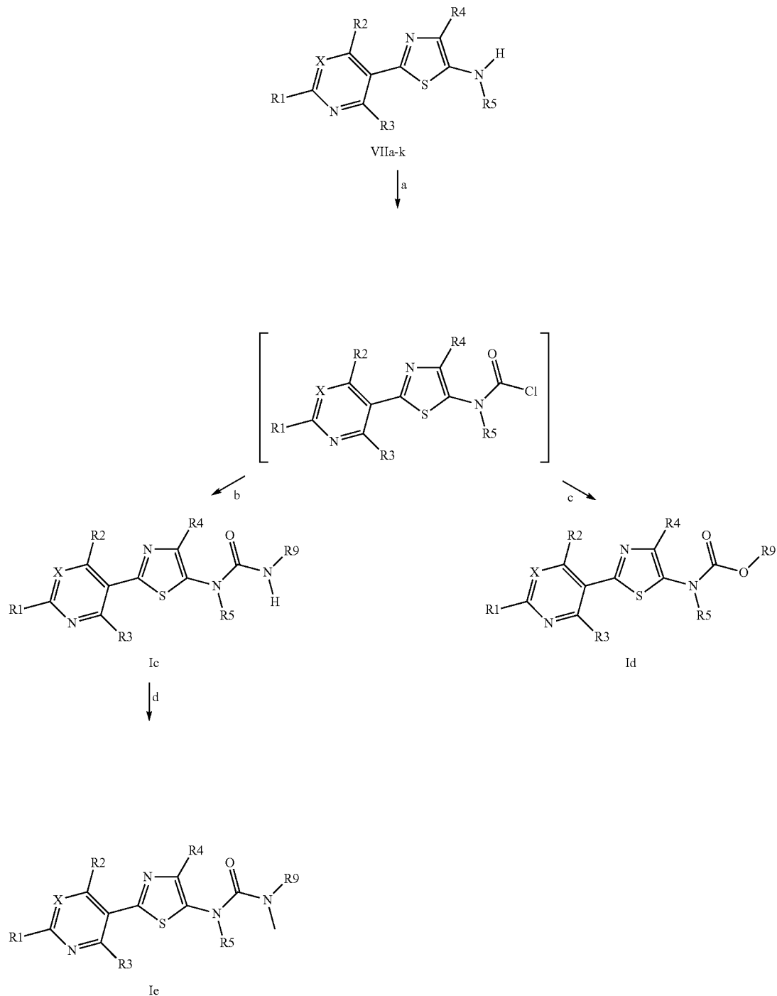
Scheme VI
