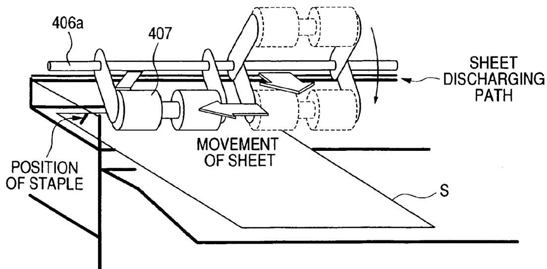
FIG. 10C
