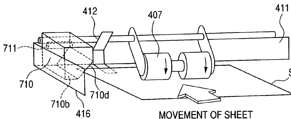
FIG. 31C
