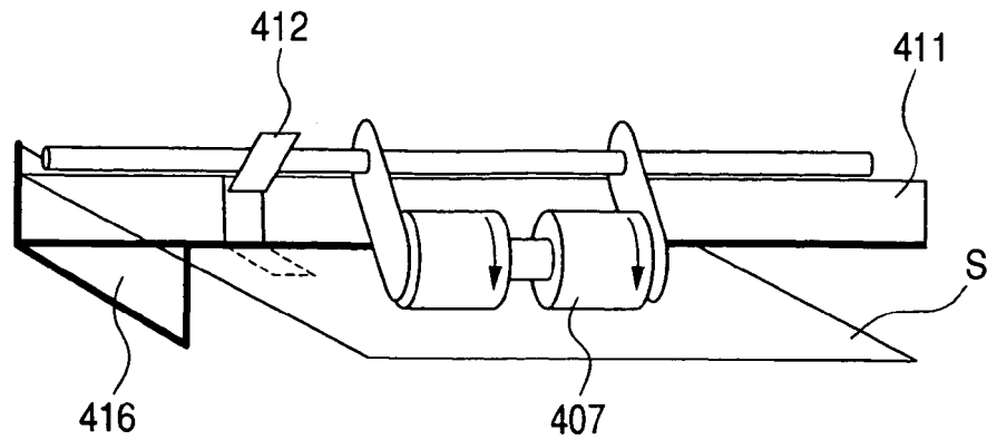
FIG. 12A
