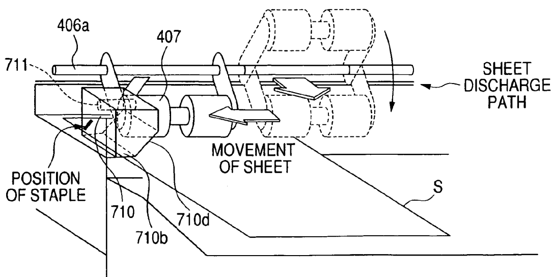
FIG. 31C
