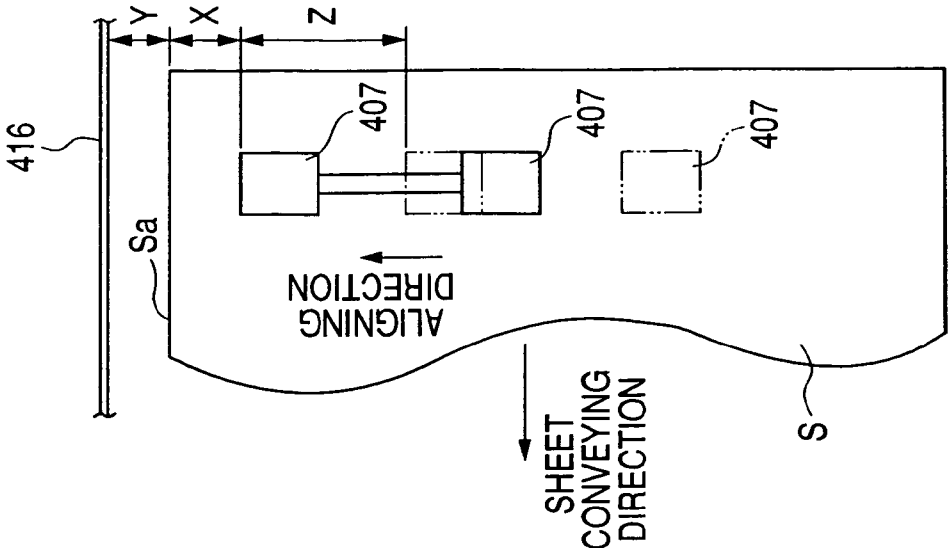
FIG. 22C
