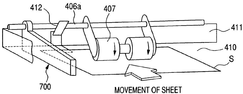
FIG. 24B
