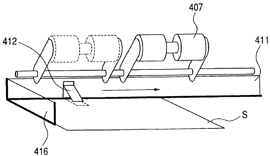
FIG. 11B
