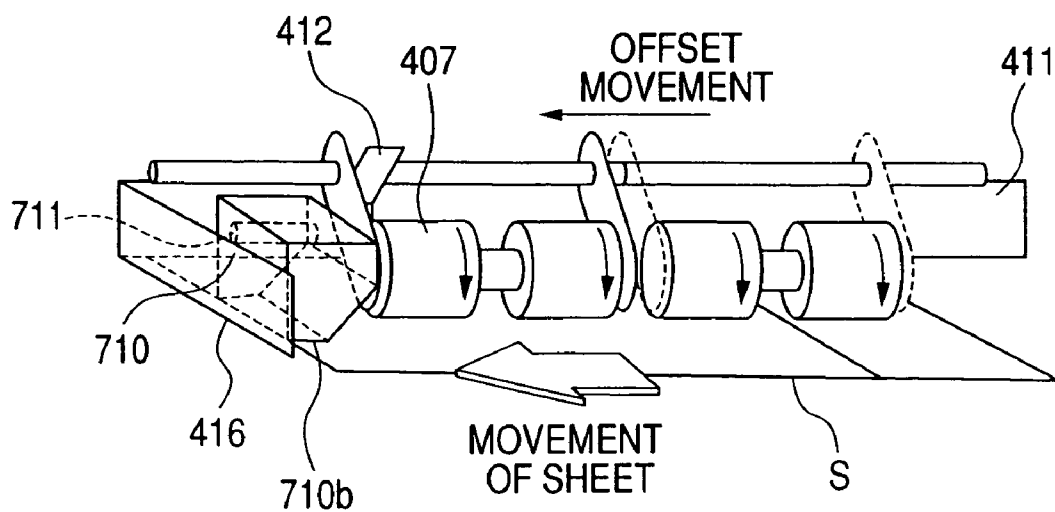
FIG. 33B
