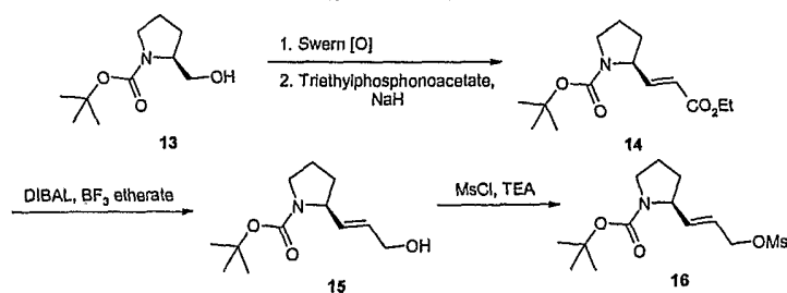
Scheme VI
