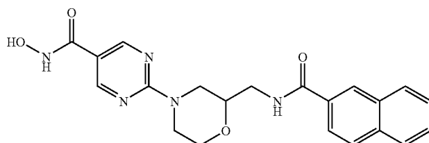
Co. No. 9; Ex. [B9]; mp. 246° C.
