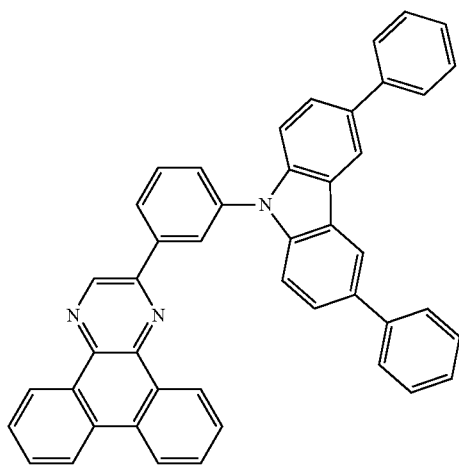
2mCzPDBq-III
