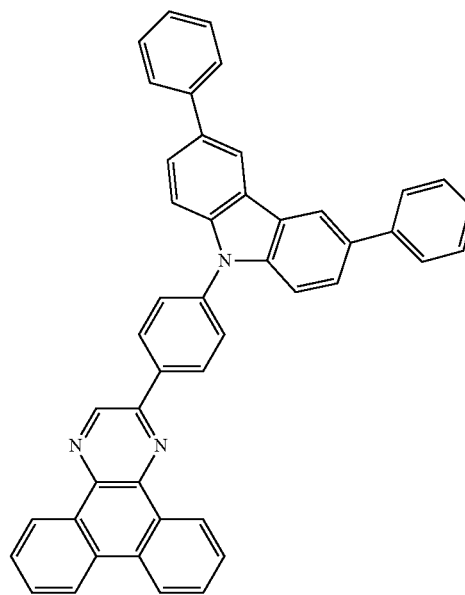
2CzPDBq-III
