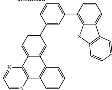
7mDBTPDBq-II
