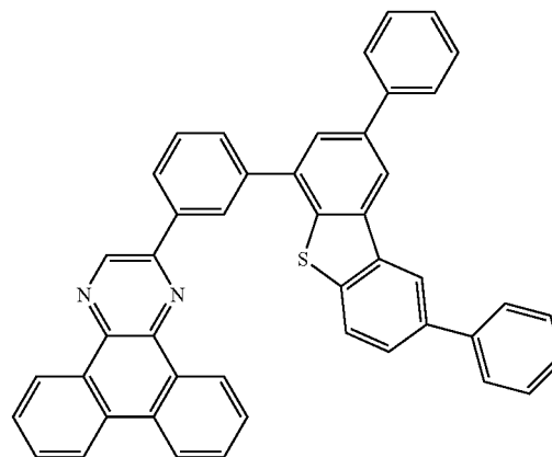
2mDBTPDBq-III
