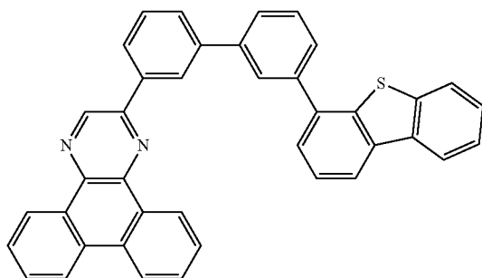
2mDBTPDBq-II
