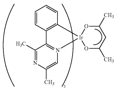
Ir(mppr-Me) 2 acac
