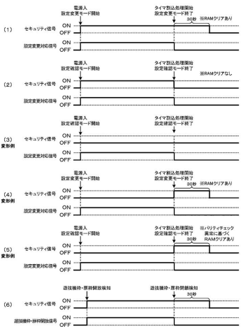
【図 21-40】 セキュリティ信号及び設定変更対応信号の出力期間
