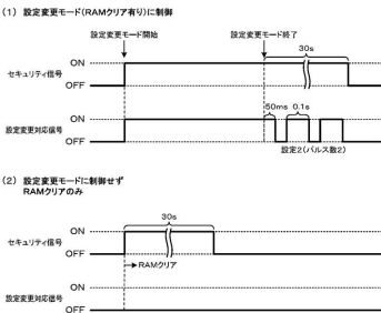
【セキュリティ番号の出力期間】
