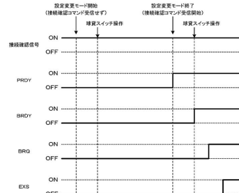
【図 21-28】 第2の球貸制限方法
