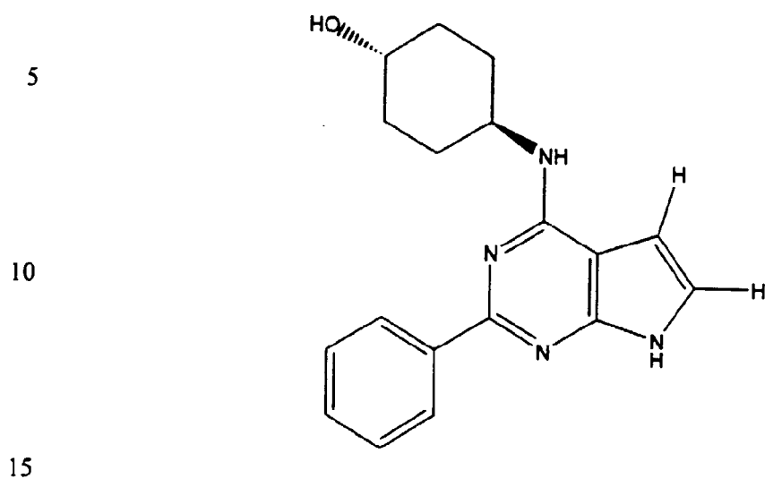
(Compound 1318-a)
