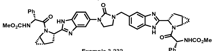
Example 3-232
