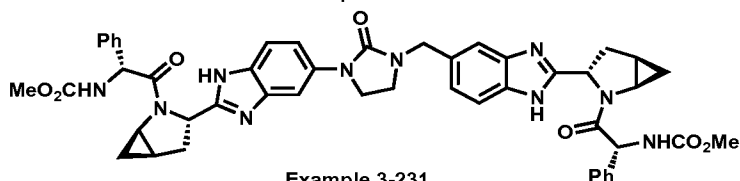
Example 3-231
