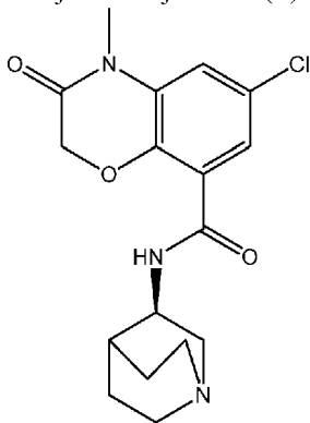
(R)-I
