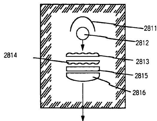
Fig. 18(D) Light Source Optical System
