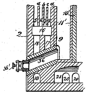
Section V-V
