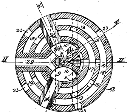
Section E-F Fig. 7
