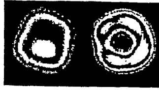
Laguerre-Gaussian mode VCSEL:
