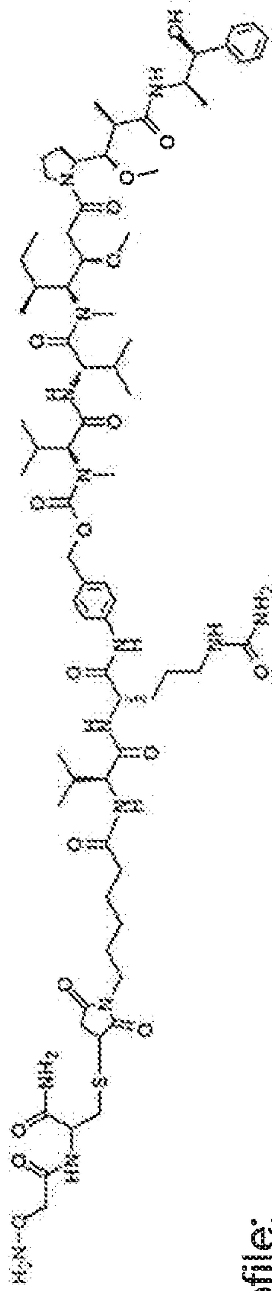
Aminoxy MC-VC-PABC-MMAE
