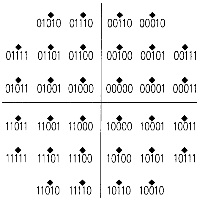
FIG. 12d 5 BITS PER BAUD
