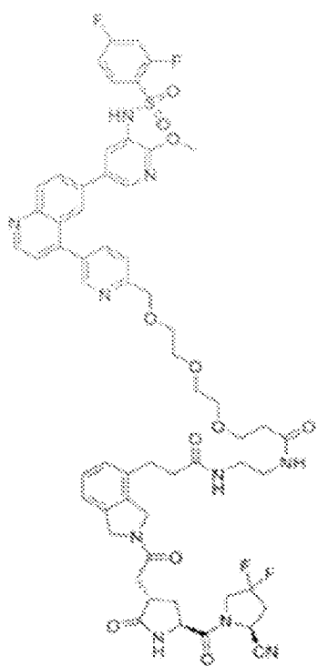
FAP5-PI3Ki-NR
