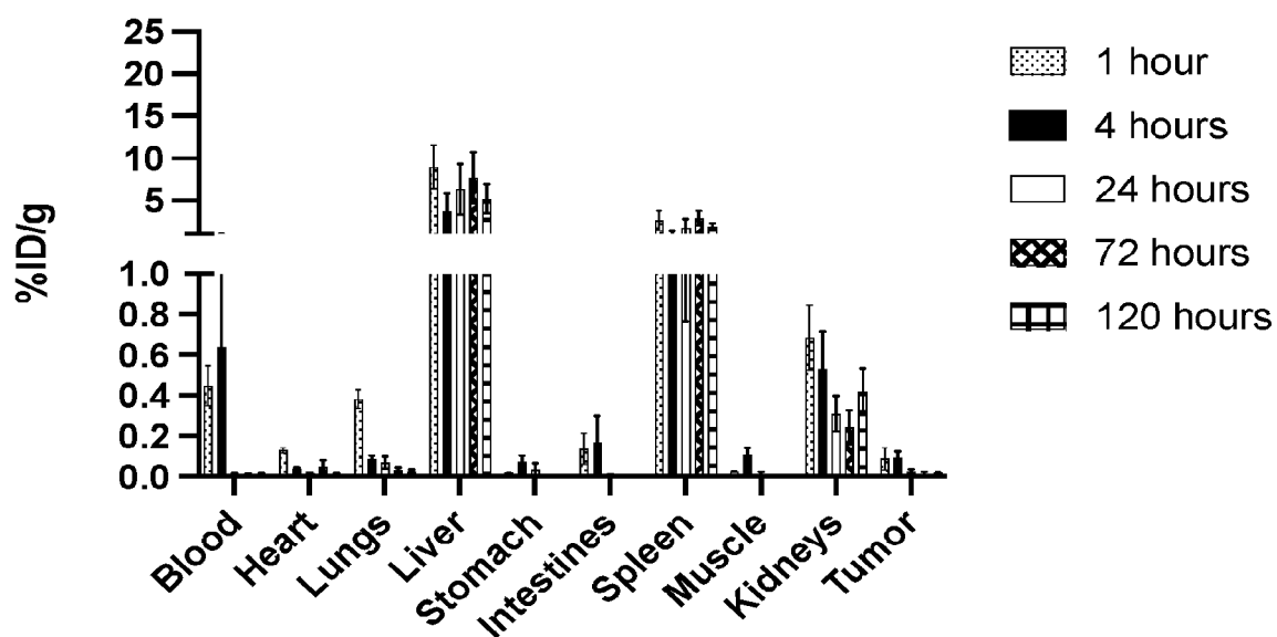
Fig. 8A Biodistribution of ^{177}\text{Lu} -FAP-3000
