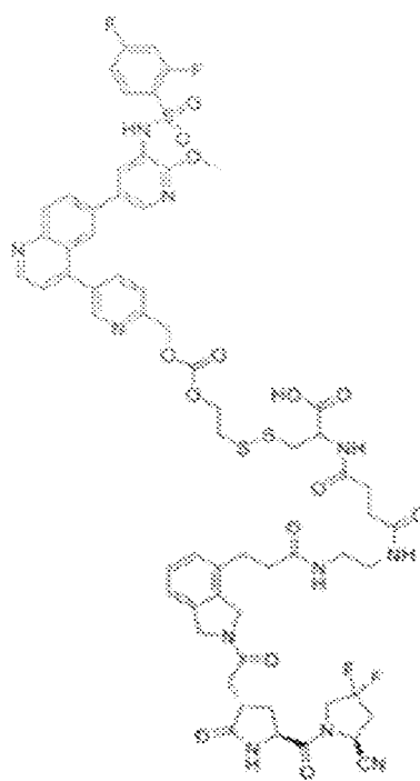
FAP5-PI3Ki-R
