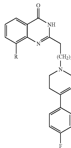
R = Cl R = Me
