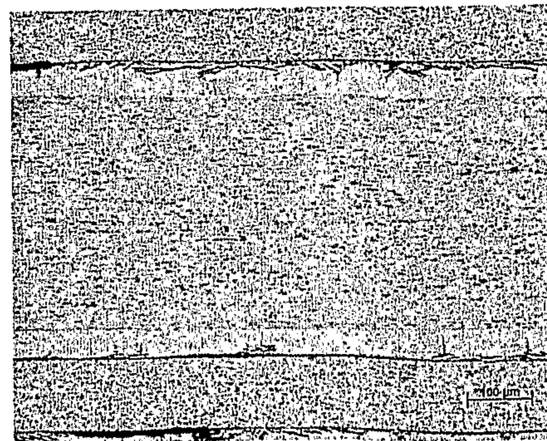
8% Stretch FIG. 7o
