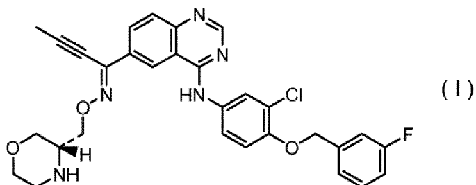
(Chemische Formel 2)
