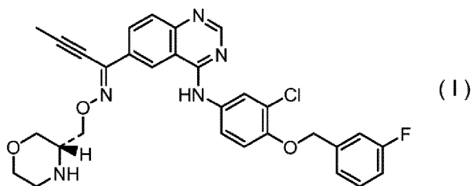
(Chemische Formel 2)
