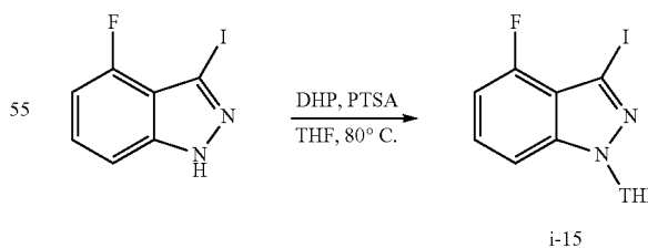
Scheme i-15
