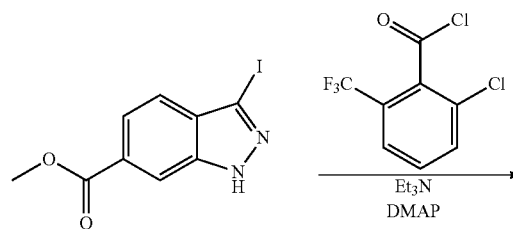
i-14c
