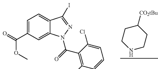
i-14c
