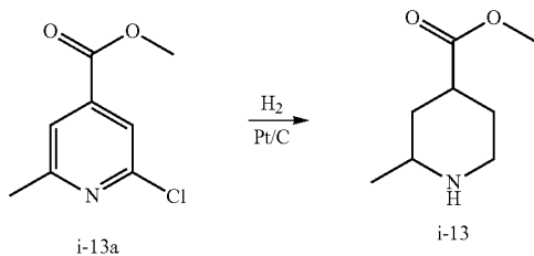
i-13a
