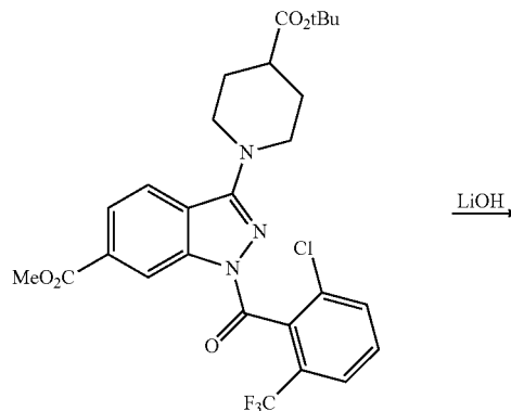
i-14e
