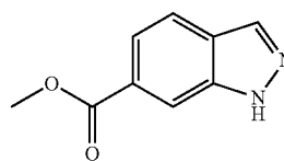
i-14b
