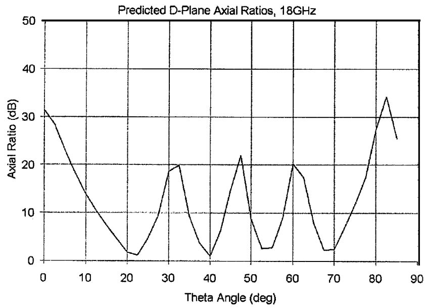
Fig. 10a (Pyramidal design)
