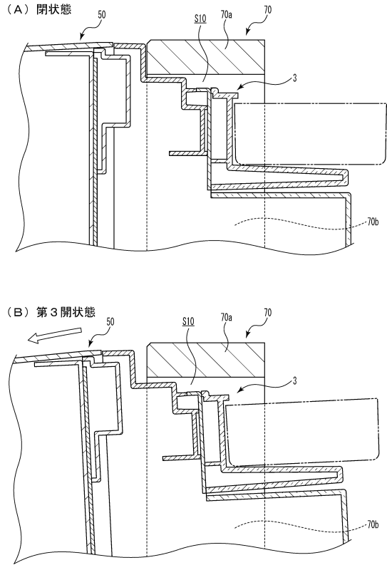
遊技機用枠と外枠 (遊技盤ユニットの上部と上板の内面)
