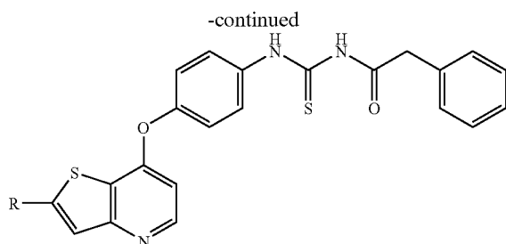
258a: Example 215
