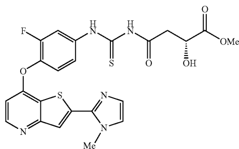
220f: Example 199
