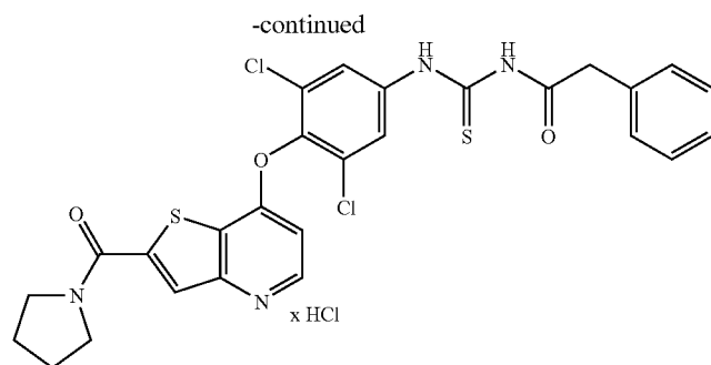
143: Example 100
