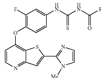
220a: Example 194
