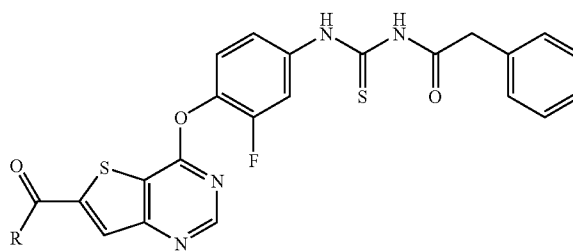
26a: Example 22
