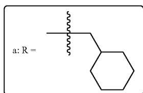
220f: Example 199
