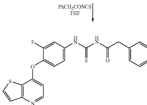
170a: Example 133
