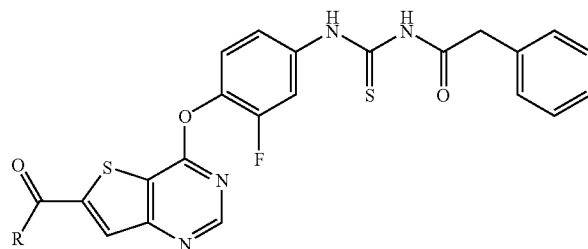
26f-l: Examples 142–148
