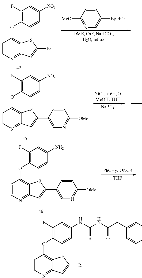
47a: Example 49
