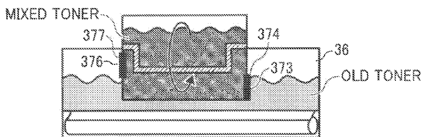
FIG. 6D
