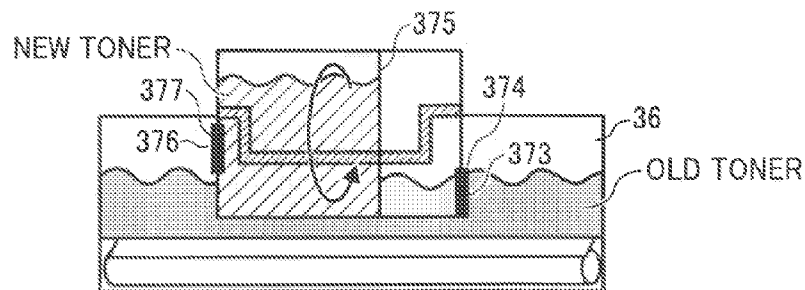
FIG. 6C
