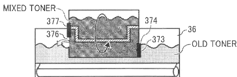
FIG. 6E
