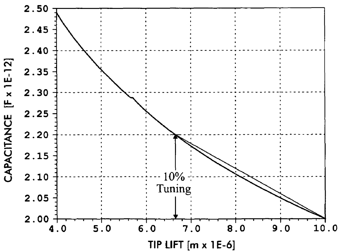
FIG. 56
