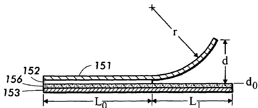
FIG. 55
