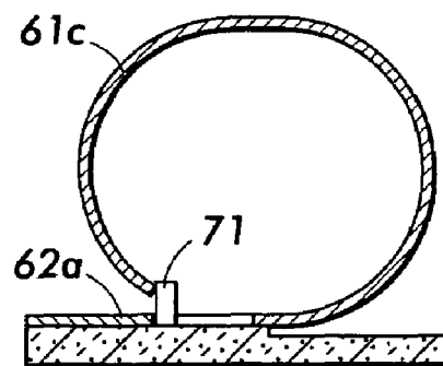
FIG. 36B
