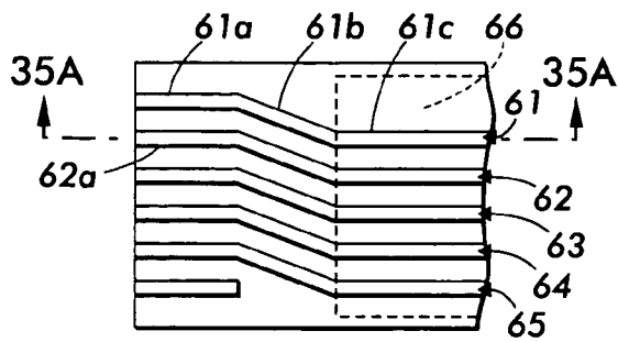
FIG. 35B
