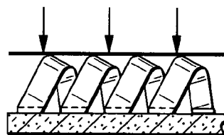
FIG. 39D
