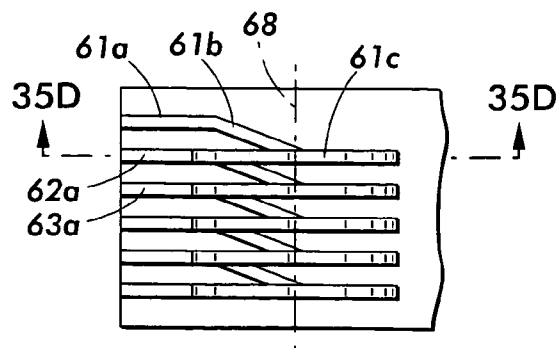
FIG. 35E
