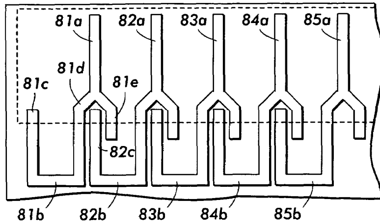
FIG. 40A
