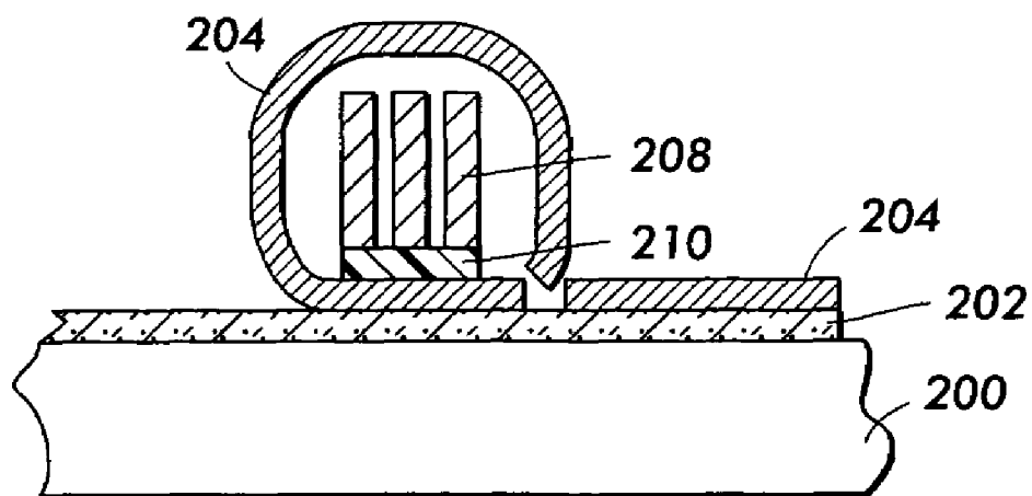
FIG. 46B
