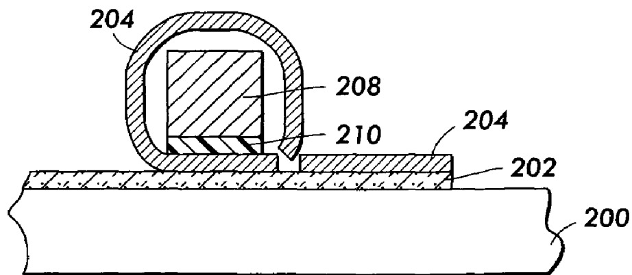
FIG. 45B
