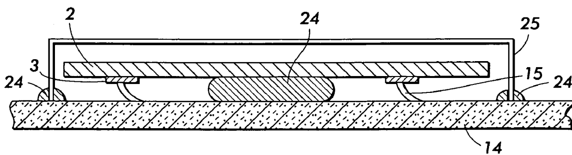
FIG. 27
