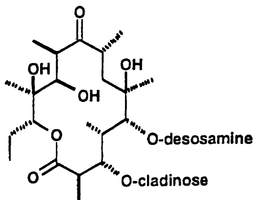
Erythromycin A
