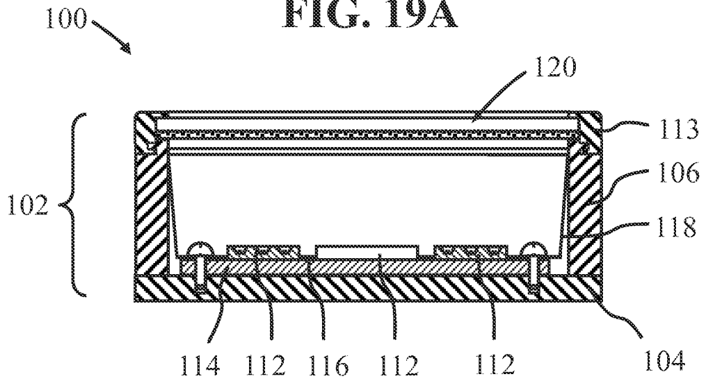
SECTION A-A
