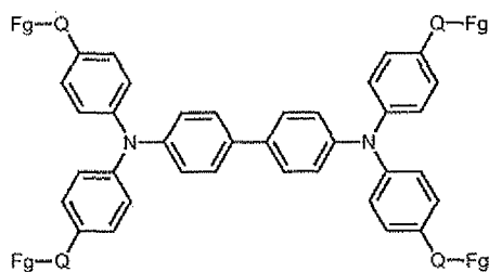
tetraaryl/biphenylenediamine (TBD) cores
