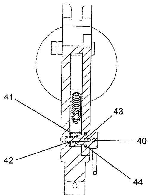
SEÇÃO B-B
