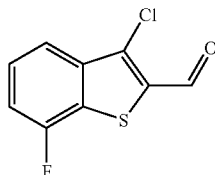
\text{C}_9\text{H}_4\text{ClFOS} Exact Mass: 213.97
