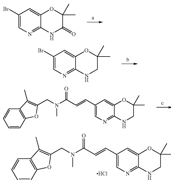
Scheme 19.
