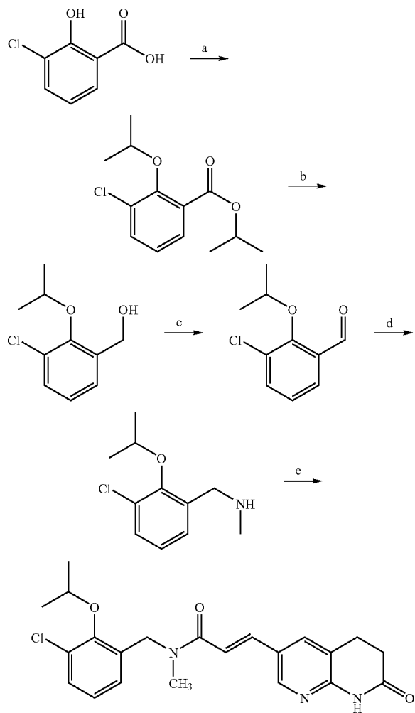
Scheme 23.
