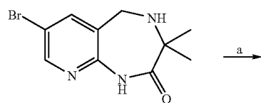
Scheme 14.
