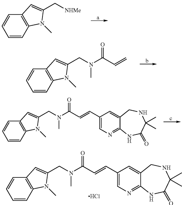
Scheme 16.
