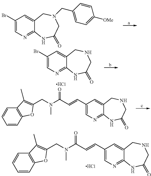
Scheme 17.
