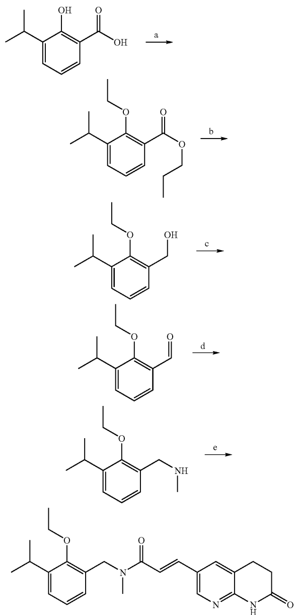
Scheme 25.
