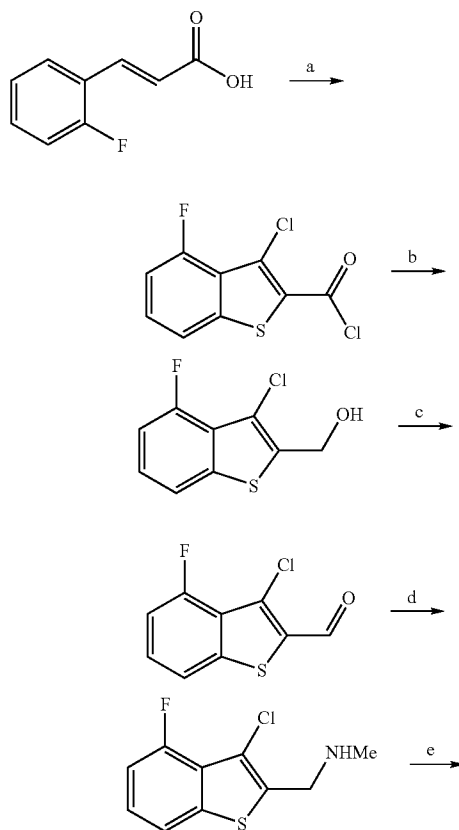
Scheme 27.
