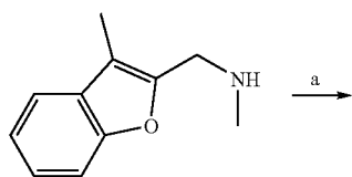
Scheme 26.
