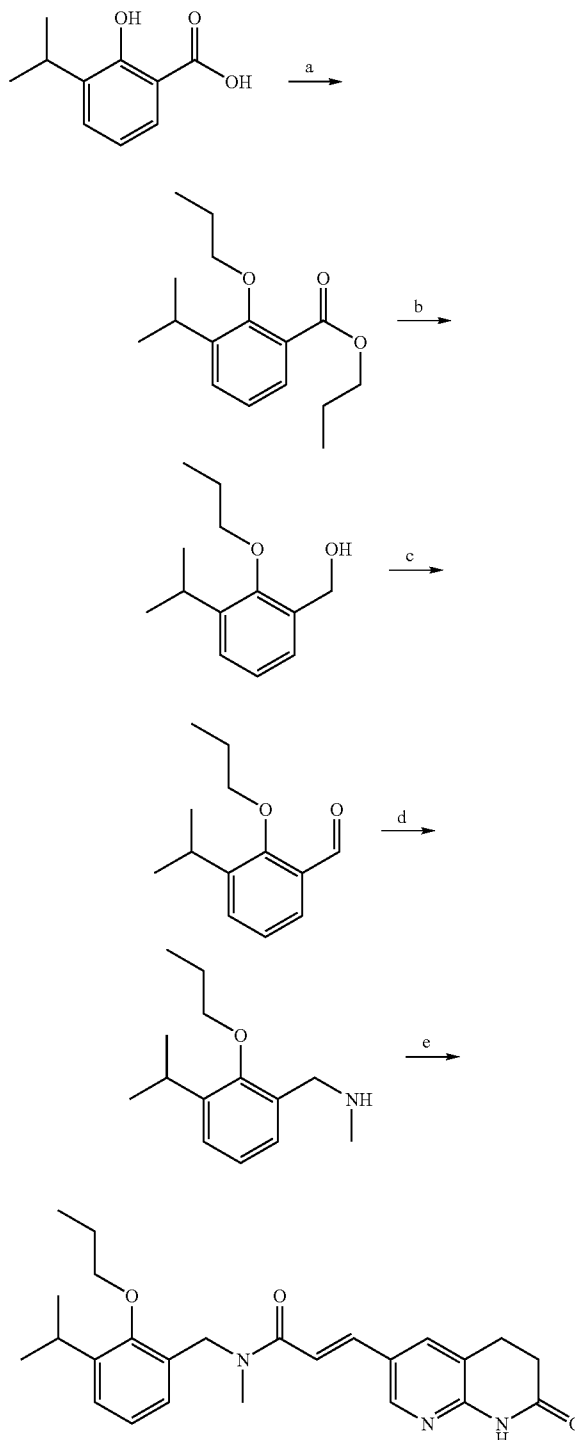
Scheme 24.
