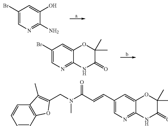
Scheme 18.
